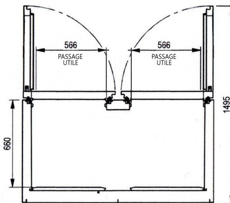
DESSUS
